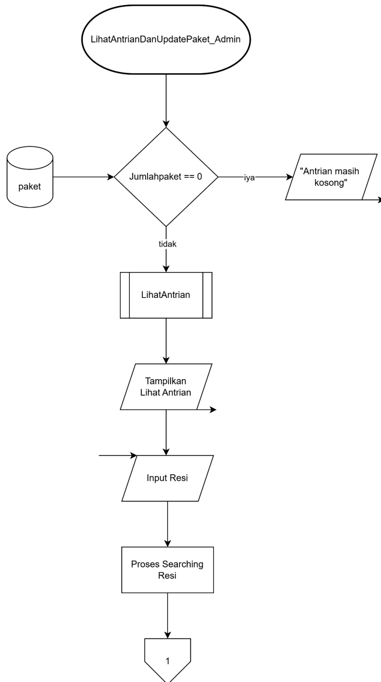
Gambar 15.1 Flowchart Lihat Antrian dan Update Paket Admin (1)
