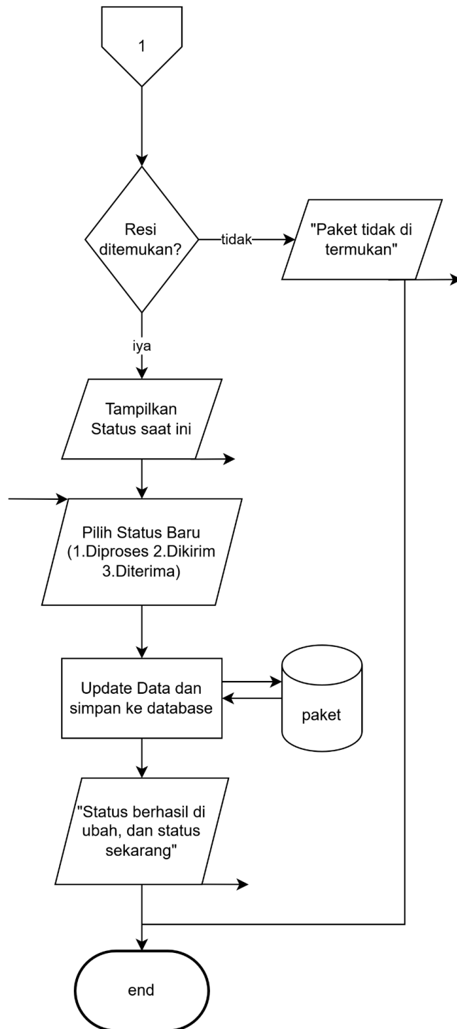
Gambar 15.1 Flowchart Lihat Antrian dan Update Paket Admin (2)
